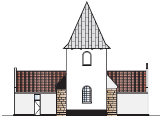
⊕ FAÇADE MOD VEST mål 1:175
