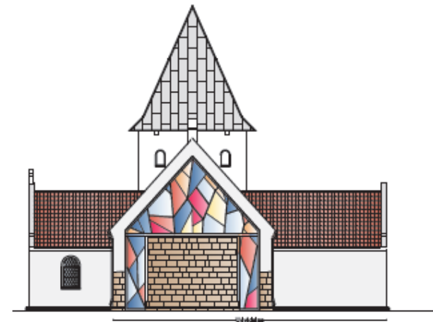
⊕ FAÇADE MOD ØST mål 1:175
